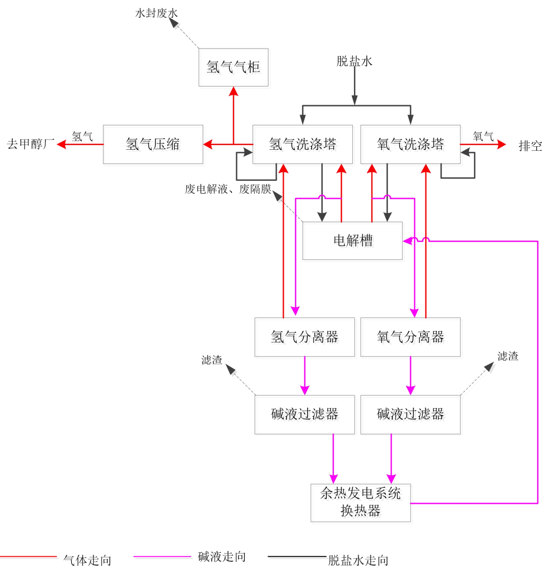
图 3.3-3 电解水制氢工艺流程及产污节点图
