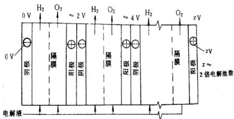
图 3.3-2 电解槽结构图
