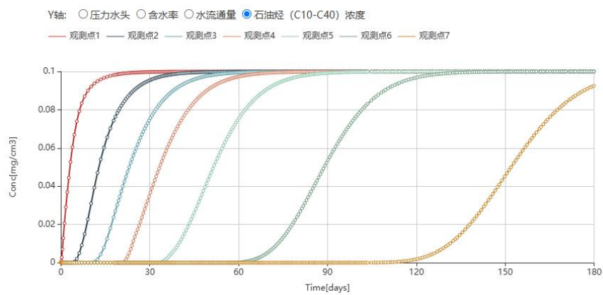
图5.7-2 不同深度处污染物浓度曲线图
