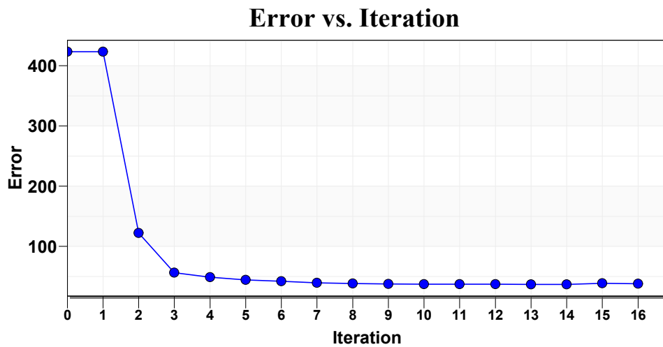
图 5.4-8 迭代次数和总体误差曲线
