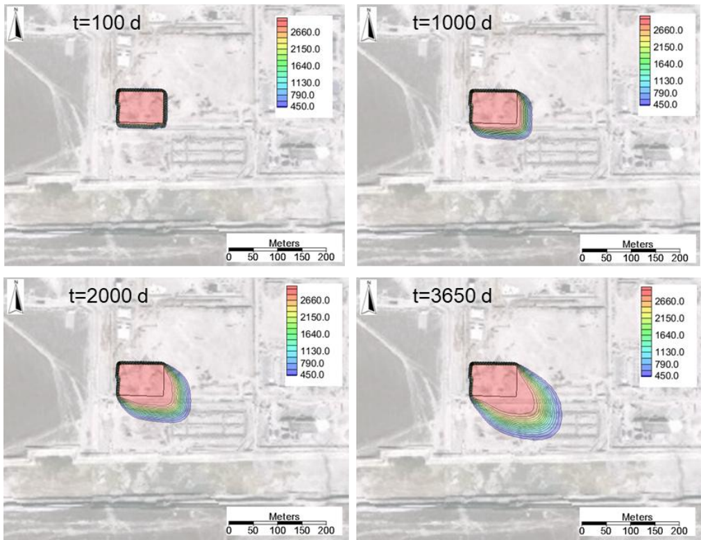
图 5.4-11 运营期 TDS 污染物不同时间污染运移范围
