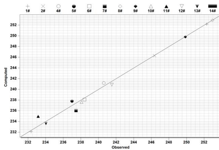
图 5.4-11 观测水位和模拟水位对比图
