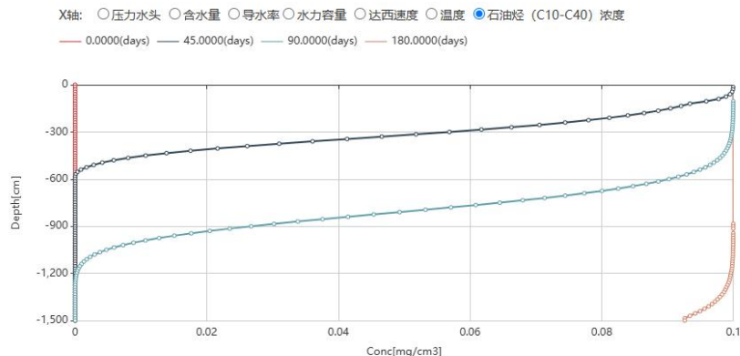
图 5.7-3 污染物在不同时段沿土壤迁移情况图
