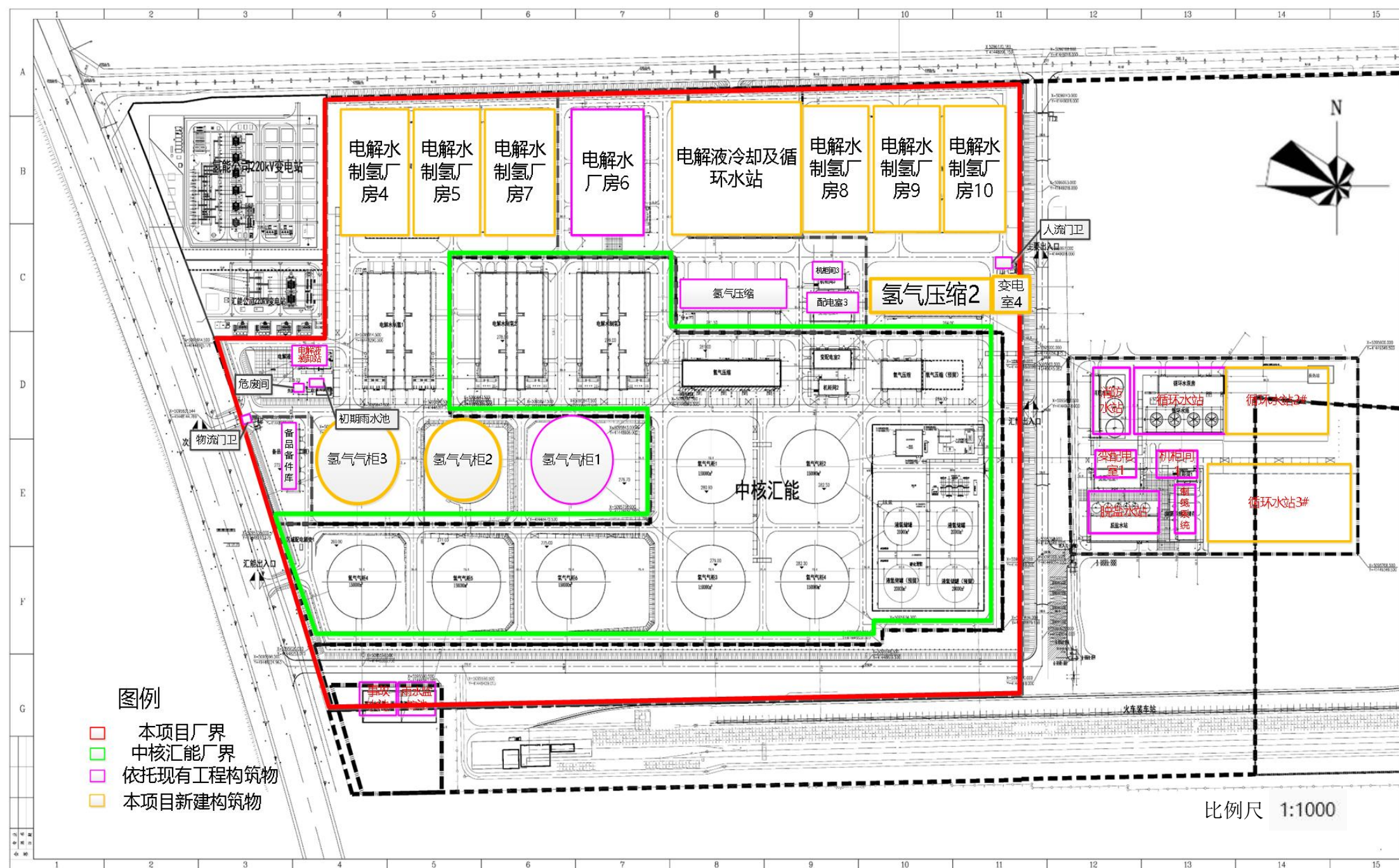
图 3.2-3 本项目总平面布置图
