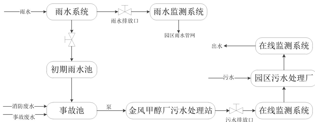
图 6.6-2 事故废水防范和处理流程示意图
