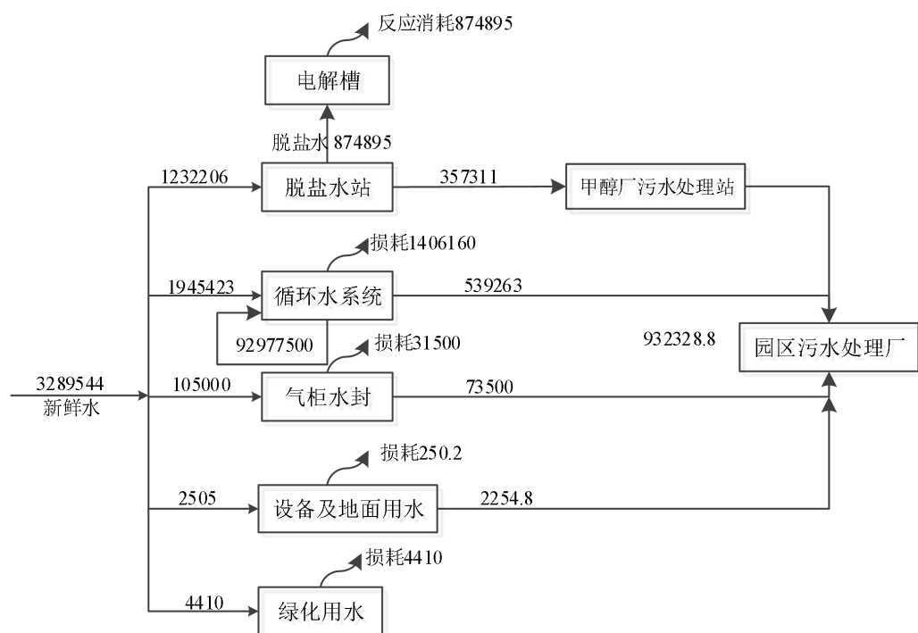
图 3.2-4 全厂水平衡图（单位 m³/a）
