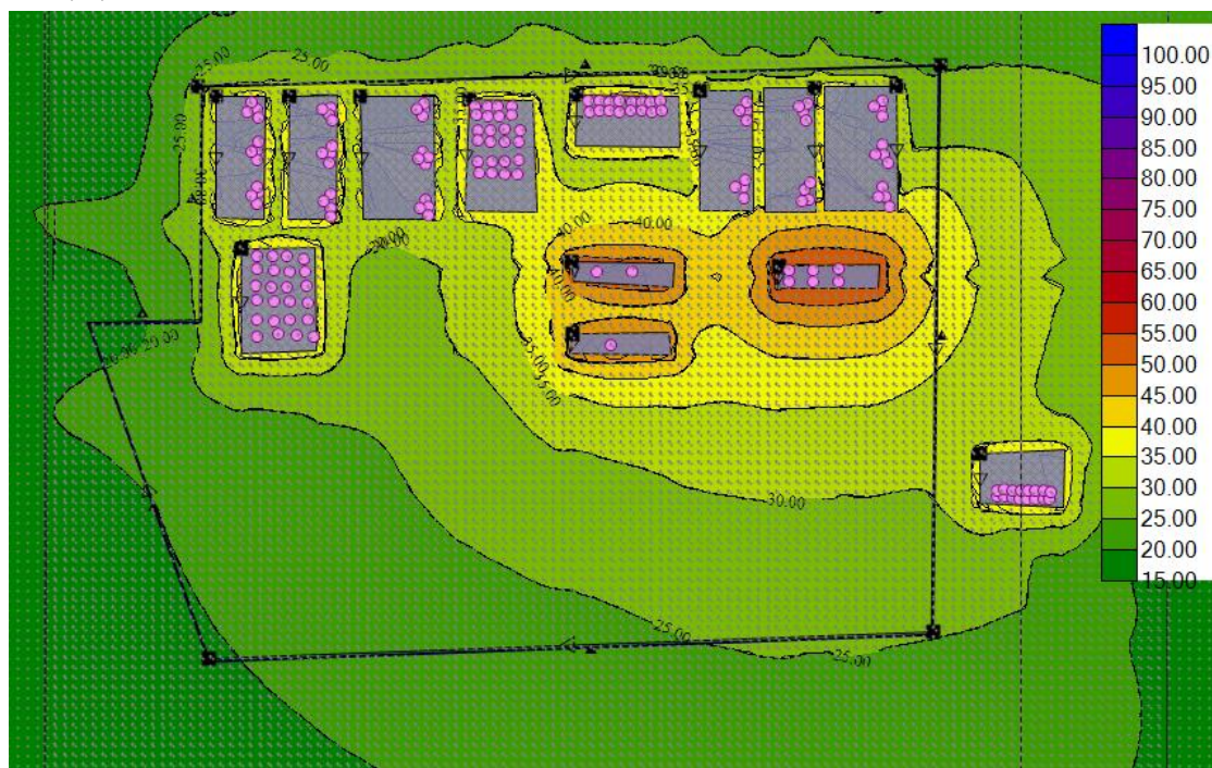
图5.5-1 厂界及噪声预测结果示意图 单位：dB(A)
