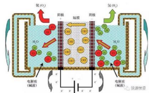
图 3.3-1 电解槽工艺图
