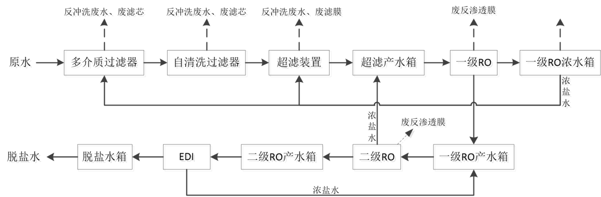
图 3.3-5 制备脱盐水工艺流程及产污节点
