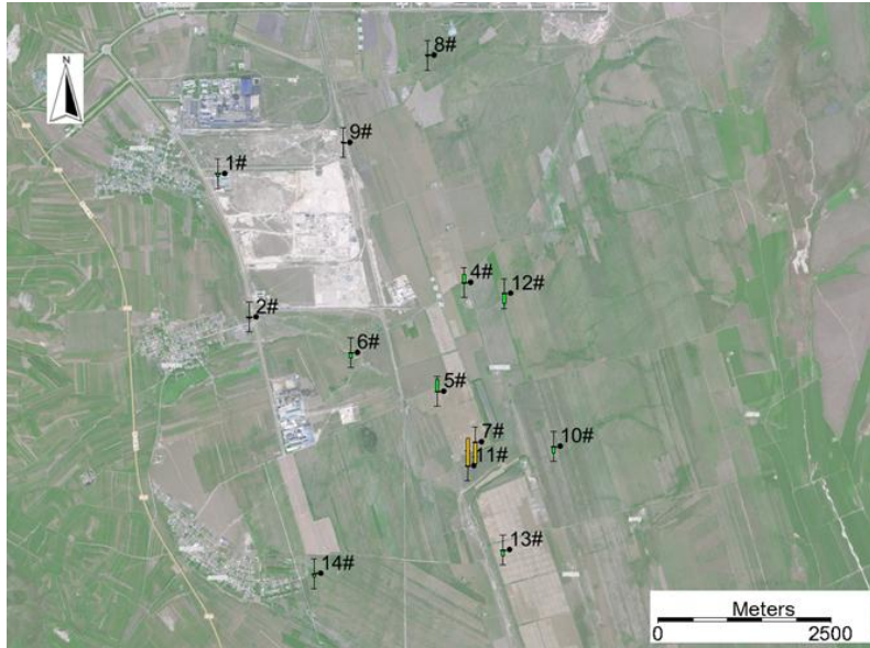
图 5.4-10 项目区内观测水位和模拟水位误差棒分布
