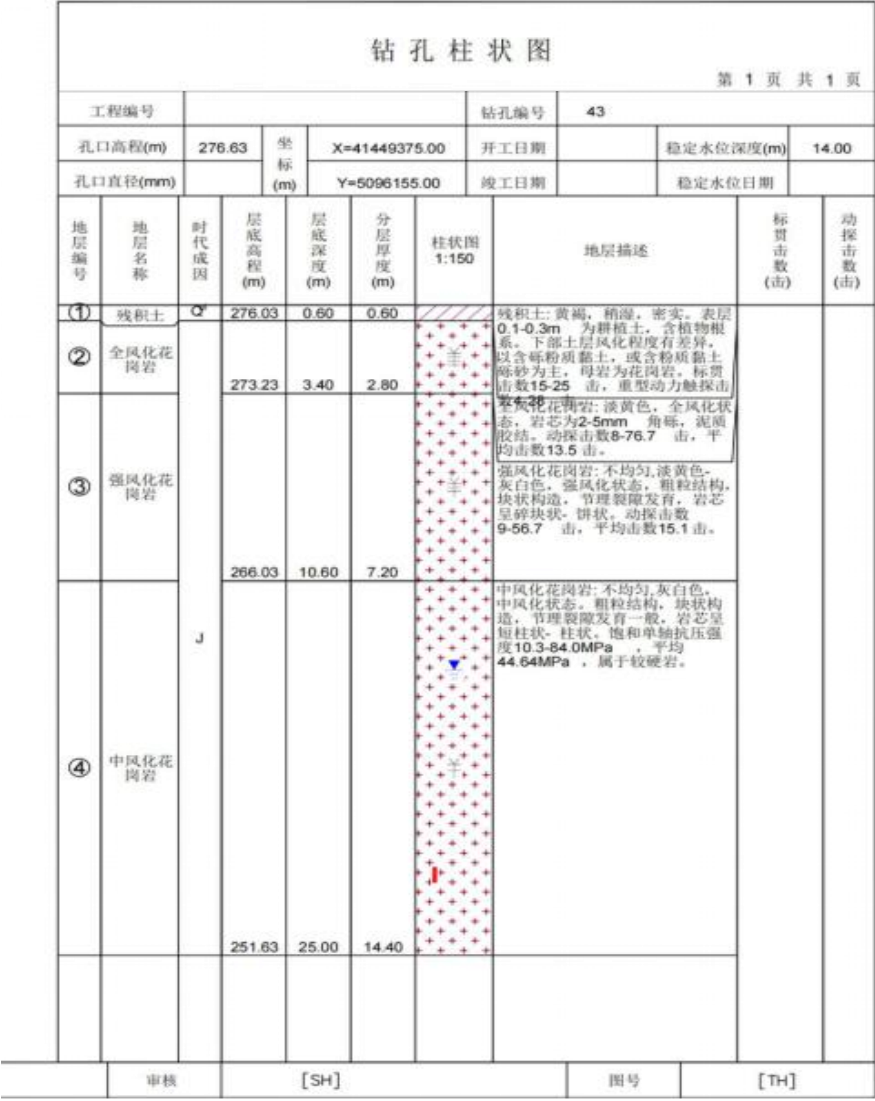
图 5.4-5 厂区钻孔柱状图
