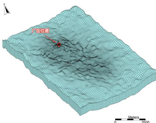
图5.4-7 数值模型网格划
