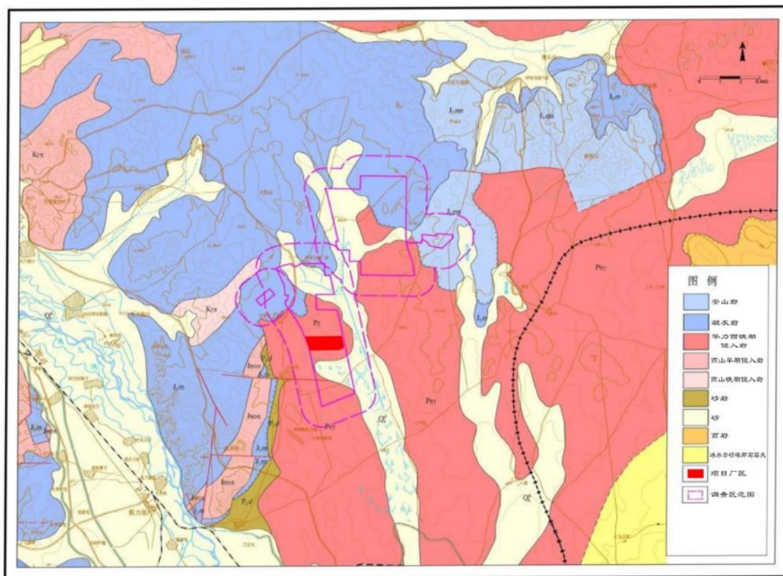
图 5.4-1 区域地质图
