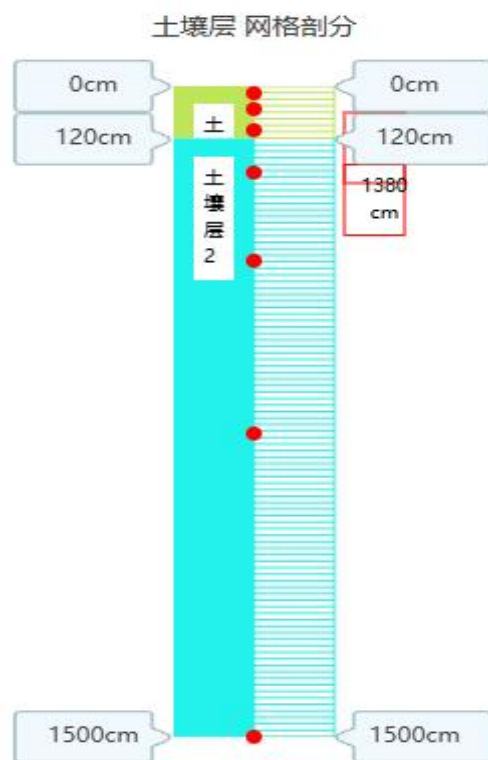
图5.7-1 厂区土壤剖面 and 观测点位置
