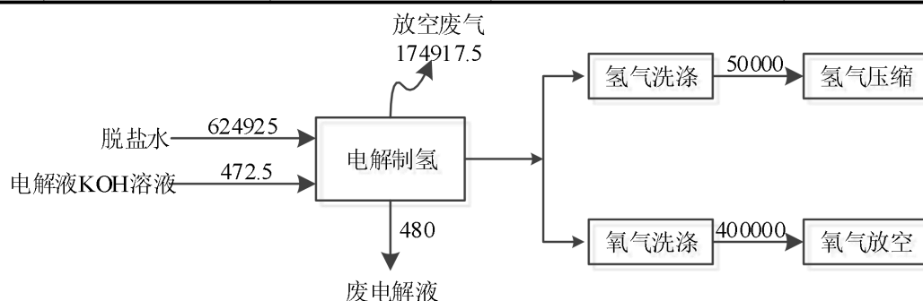
图 3.3-4 物料平衡图 单位：t/a
