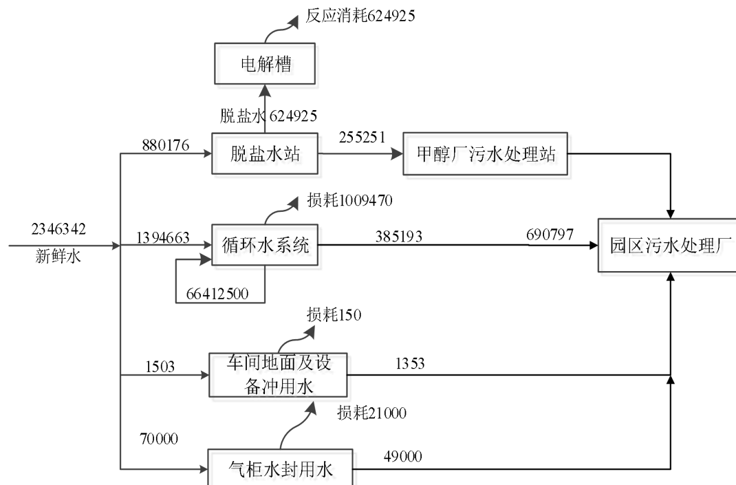
图 3.2-3 本项目水平衡图（单位 m³/a）
